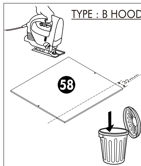
TYPE : B HOOD
