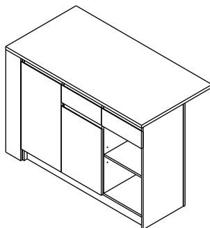
TYPE:A14 Counter Mini Island
